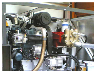
Antriebsmodul. Ansicht bei geöffneter Hecktür und entfernter Verkleidung.
