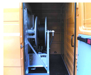
Hochdruckhaspel. Ansicht bei geöffneter Seitentür.
